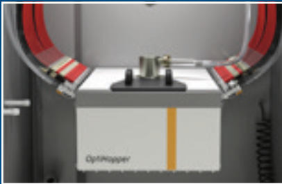
OptiHopper con inyectores OptiFlow
