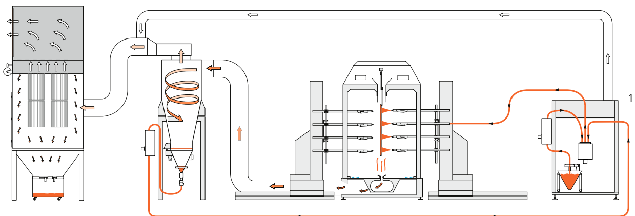
1 OptiCenter equipado con cono para bolsas de polvo fresco
